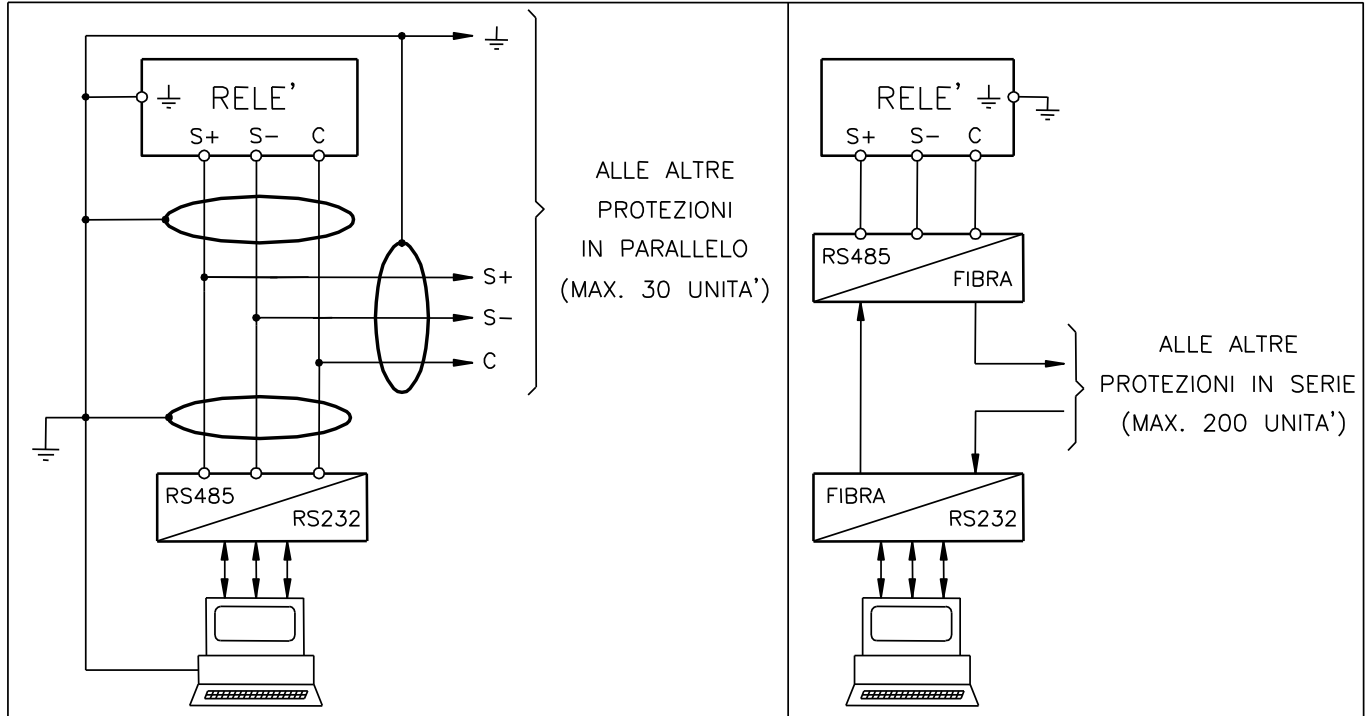
CONNESSIONE RS485
